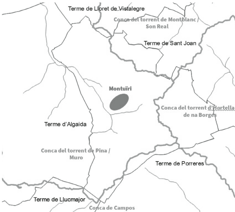
Figura 6. Croquis de la xarxa hidrogràfica principal del terme de Montuïri, límits de conques i límits de municipis. Les línies gruixades representen les divisòries d'aigües (límits de conques) i les línies negres primes, els límits de terme municipal.
