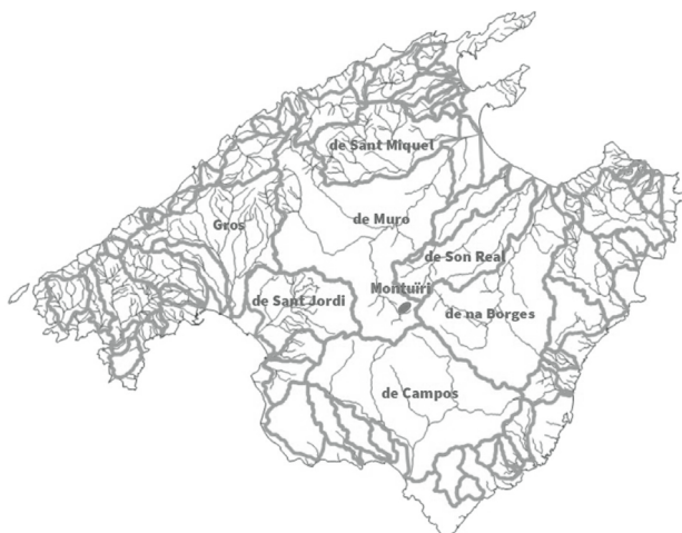
Figura 4. Conques principals de Mallorca.
