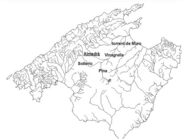
Figura 5. Ramals principals del torrent de Muro.
