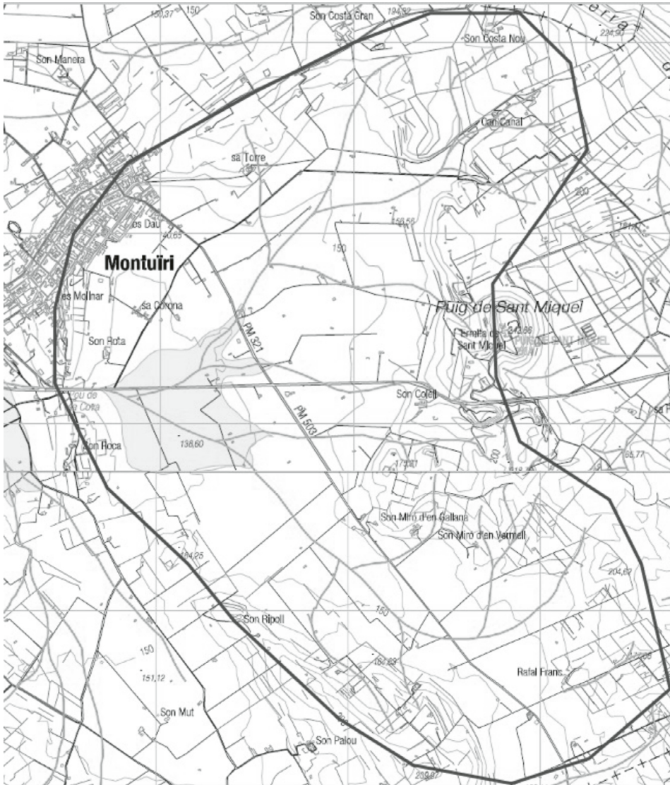
Figura 9. Detalls del límit (línia gruixada), la xarxa de drenatge i la plana d'inundació (l'antic aiguamoll) de la conca endorreica de Montuiri.
