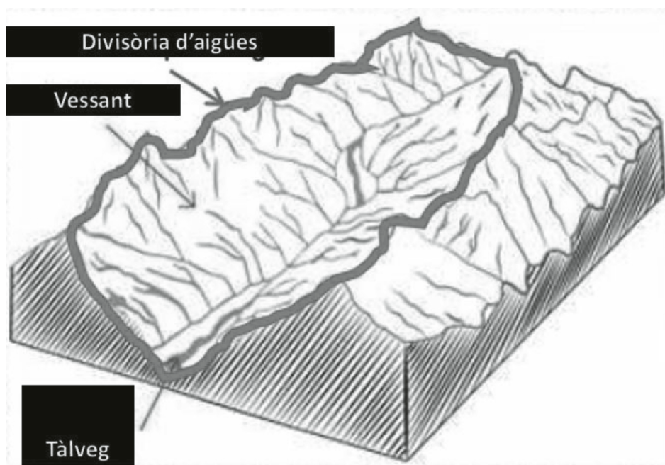
Figura 2. Divisòria d'aigües, vessant i tàlveg.
