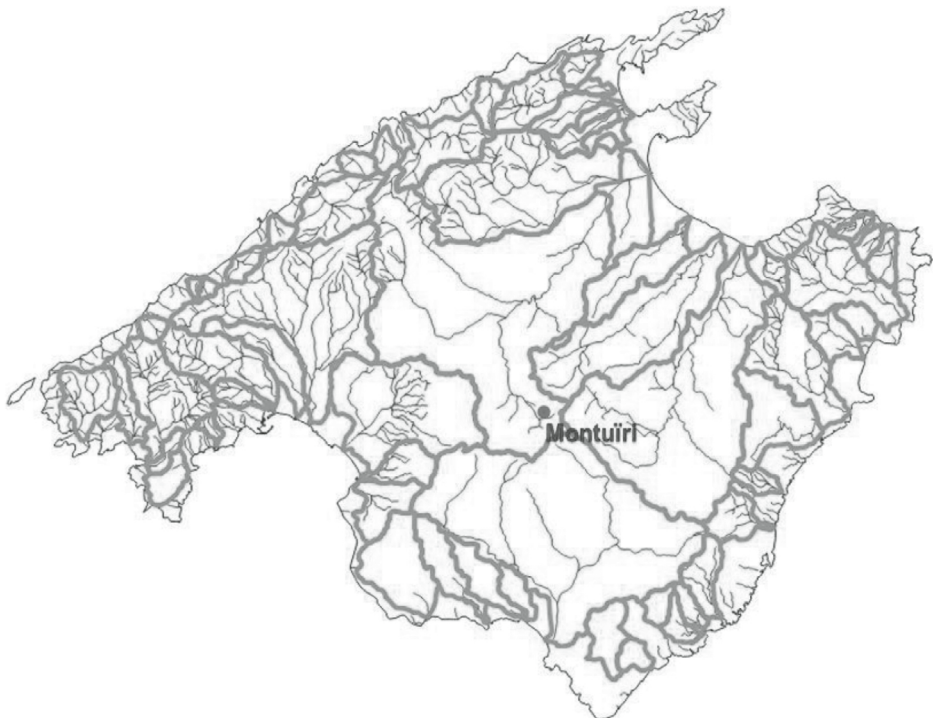
Figura 1. Límits de conques (línies gruixades) i xarxa dels torrents principals de Mallorca.
